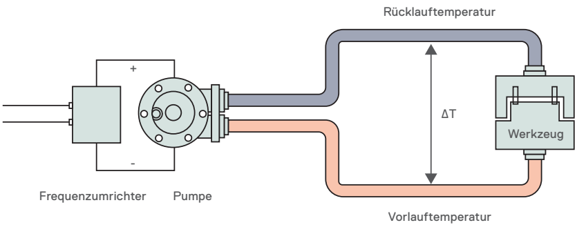
Delta-T Regelung
