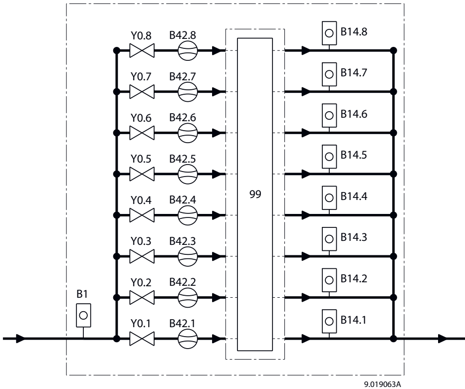
multiPulse
