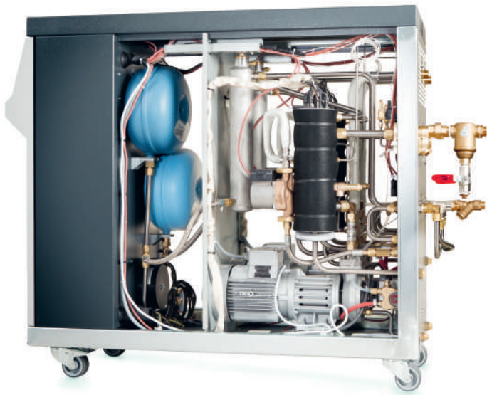
Temperiergerät P160LD/ Regelsystem RT100
